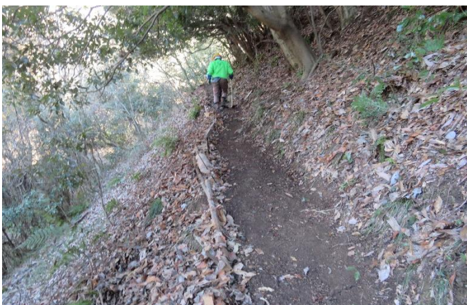
幅員を広げ、斜めの傾斜を水平に掘り下げた路
