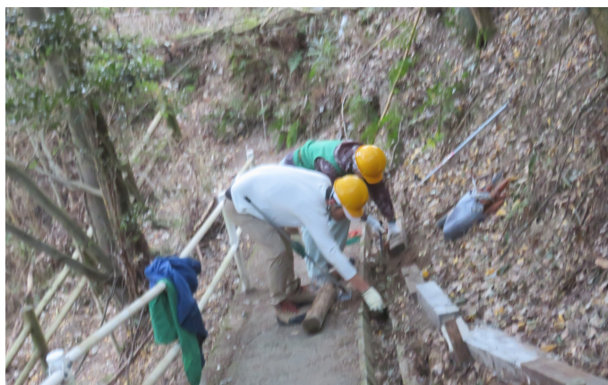
作業の様子④。角材は防腐剤を塗った木の杭と番線で固定しました。
